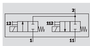
2x2/2-Wegeventil
